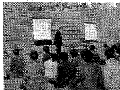
図6 時間割作成
